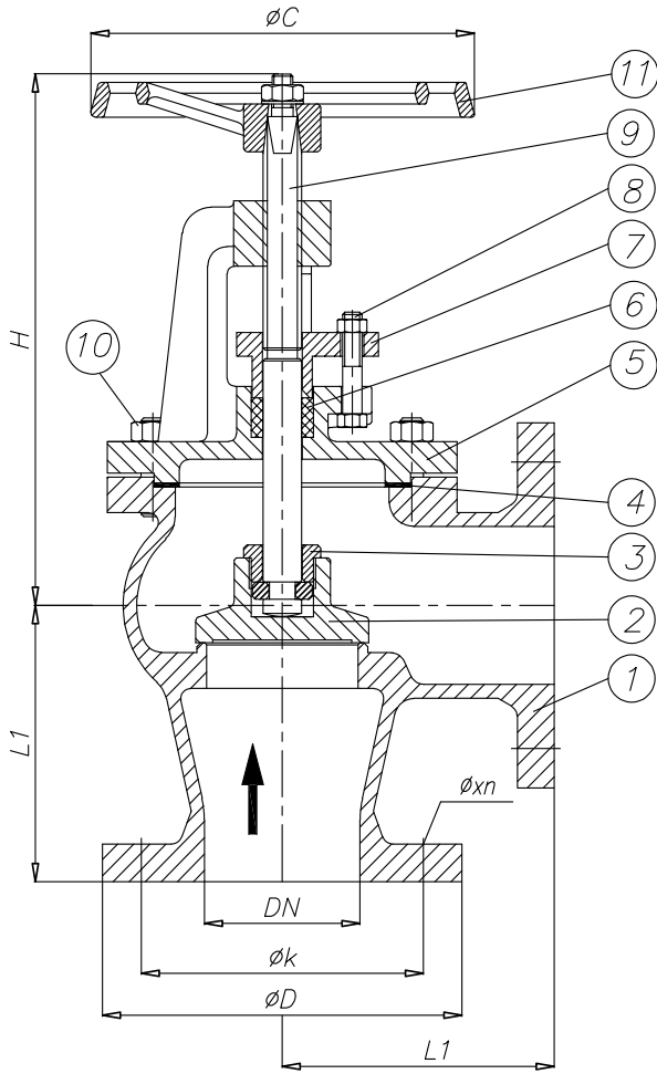
Screw Down Non Return (SDNR)
