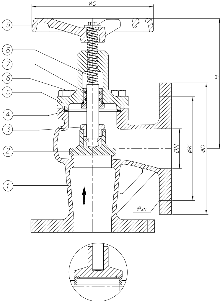
Screw Down Non Return (SDNR)
