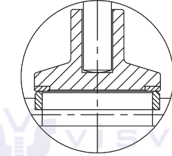
Screw Down Non Return (SDNR)
